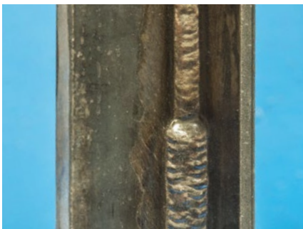
Mehrlagenschweißen – Steignaht
